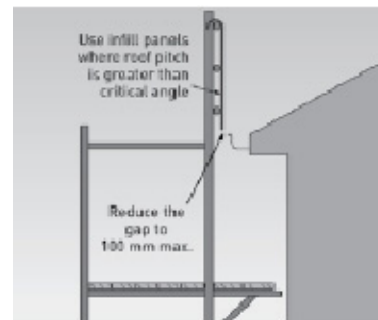
(d) Scaffolding providing guardrail protection
